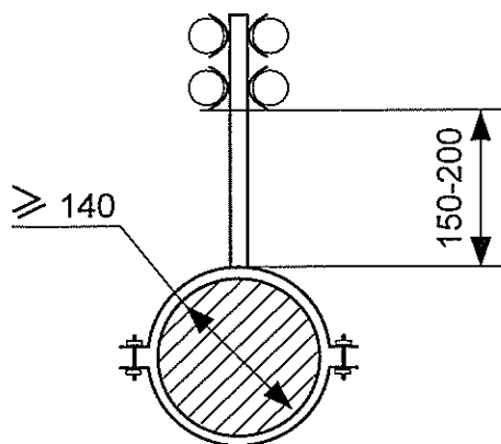
Рис. 5. Общий вид узла крепления кабеля к деревянной опоре ВЛ 0,4 кВ
