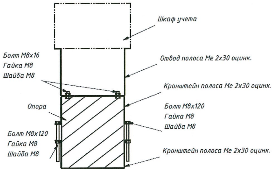
Рис.3. Общий вид узла крепления шкафа учета к опоре ВЛ 0,4 кВ
